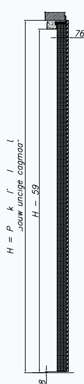
Blok kozijn
