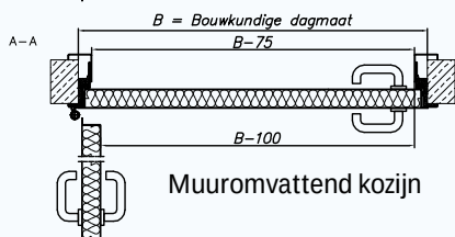
Blok kozijn
