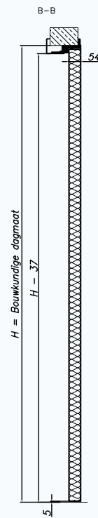
Muuromvattend kozijn
