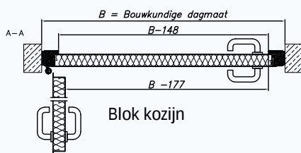
Hoek kozijn
