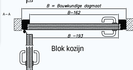
Hoek kozijn
