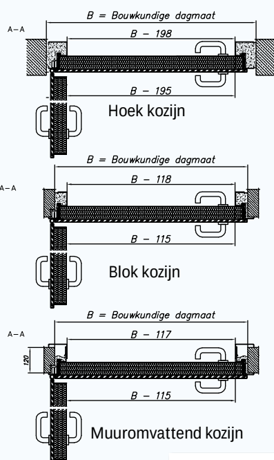
Hoek kozijn
