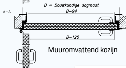
Blok kozijn
