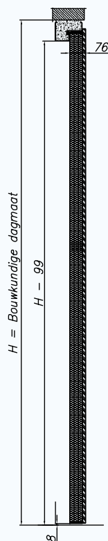
Hoek kozijn
