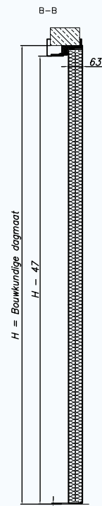
Muuromvattend kozijn
