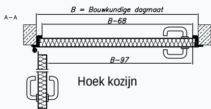
Hoek kozijn
