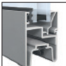
U-waarde Panoramadeur 40: 4000 x 4000 mm 4,35 W/m 2 K.
